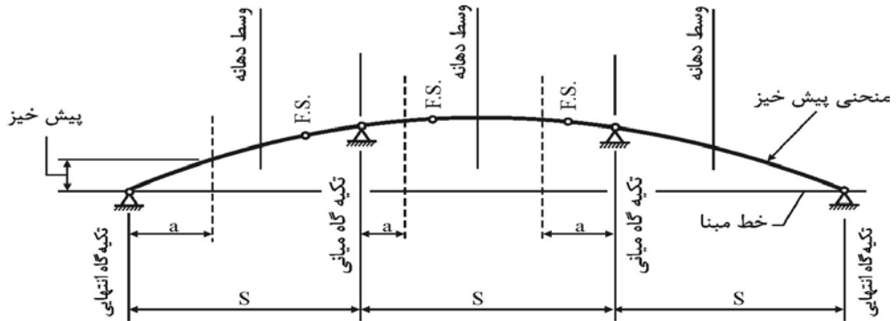
F.S. وصله کارگاهی
