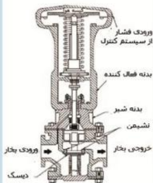
فعال کننده پنوماتیکی
