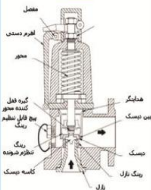
ساختار داخلی یک شیر
