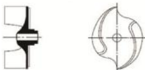
پروانه S شکل و بدون انسداد دو راهه
