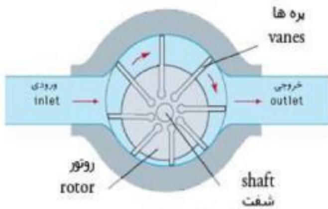
طرح کلی یک پمپ پره
