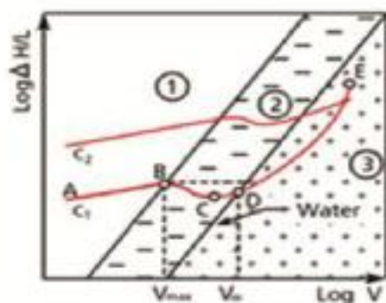
هدرفت اصطکاکی در لوله در مقایسه با سرعت و غلظت پالپ شیمیایی
