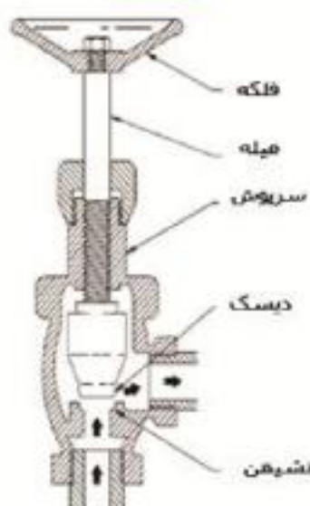
شیر کروی زاویه دار
