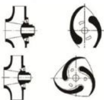
پروانه های بدون انسداد دو راهه و سه راهه
