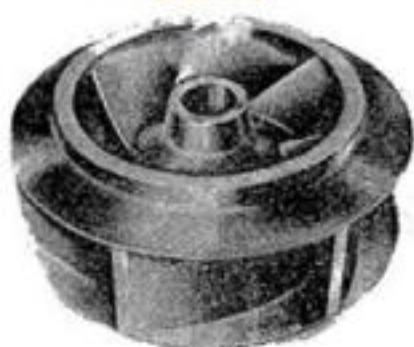
پروانه دو مکشه بسته از نوع فرانسسیس
