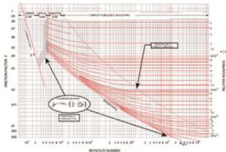
دیافراگم مودی ، فاکتور اصطکاک در برابر عدد رینولدز یکنواخت واشفته در لوله های مختلف با مقدار زبری متفاوت برای جریانات
