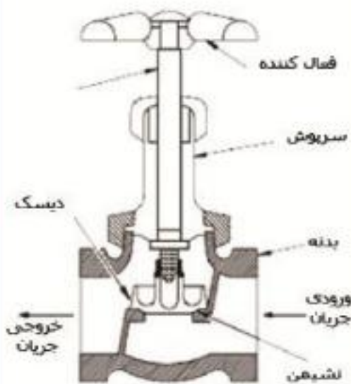
شیر اطمینان توقف کننده
