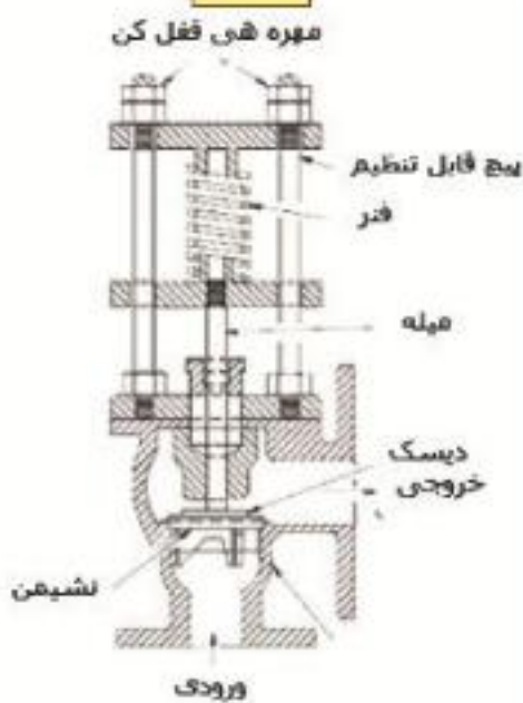
شیر فشار شکن
