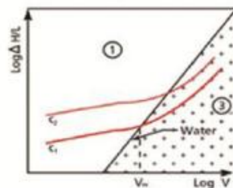
هدرفت اصطکاکی در لوله در مقایسه با سرعت و درجه پالپ مکانیکی
