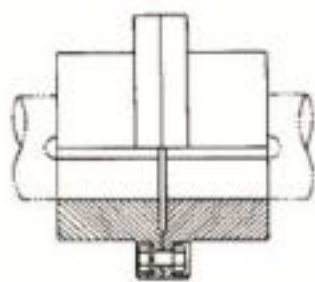
کوپلینگ بدون انعطاف فلنجی
