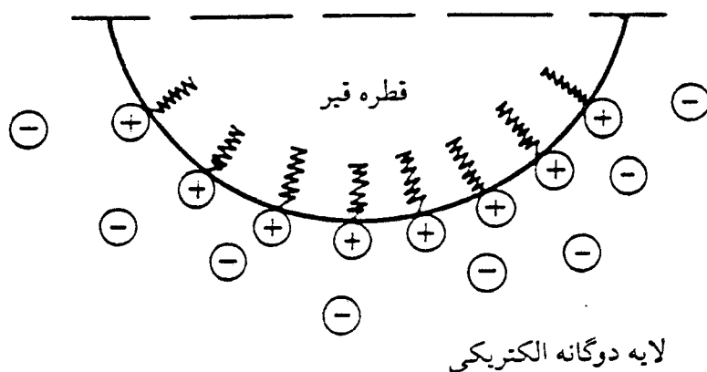
شکل ۲-۴: نمایش لایه دوگانه الکتریکی
