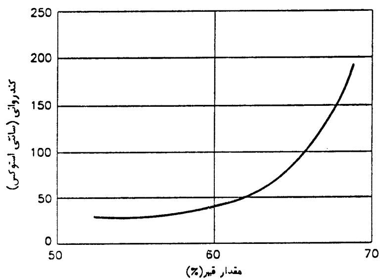
شکل ۲-۷: تغییرات کندروانی امولسیون قیری بر حسب میزان قیر [۴]
