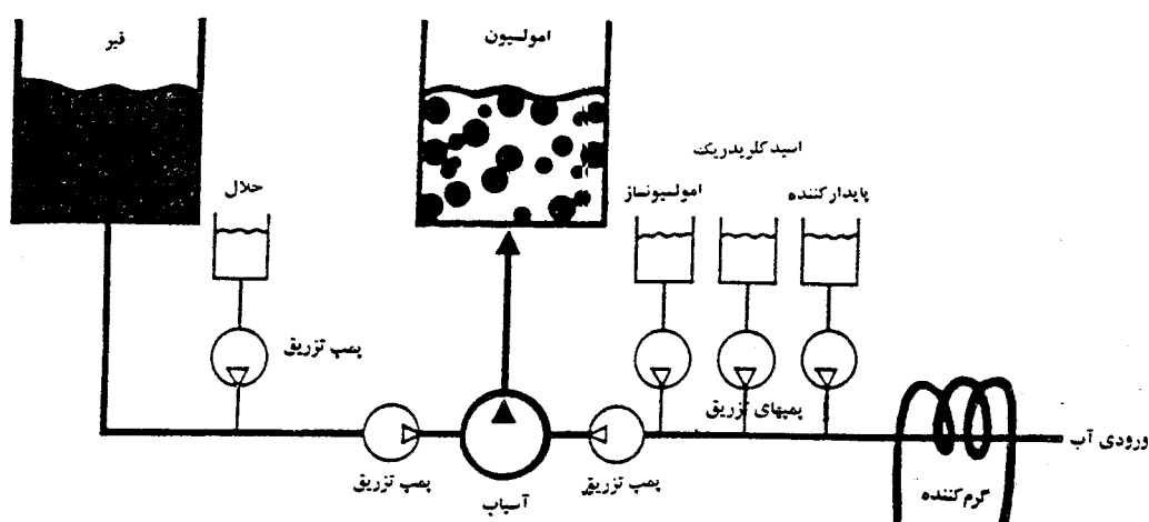
شکل ۲-۶: نموداری از کارخانه پیوسته تهیه امولسیون قیری
