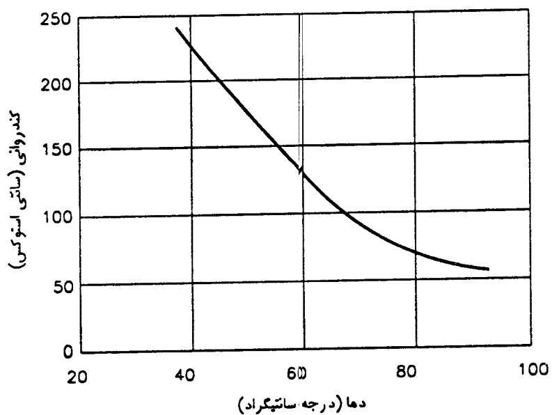
شکل ۲-۸: تغییرات کندروانی امولسیون قیری بر حسب دما [۴]
