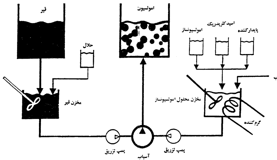
شکل ۲-۵: نموداری از کارخانه مخلوط کن پیمانهای
