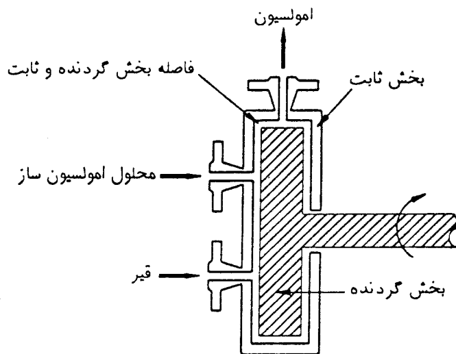
شکل ۳-۱ آسیاب کلوتیدی
