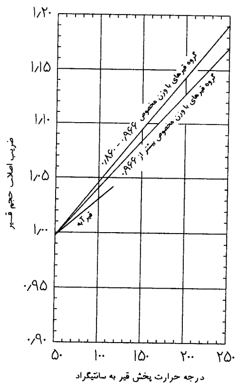
شکل ۷-۲- تعیین ضریب اصلاح حجم قیر
