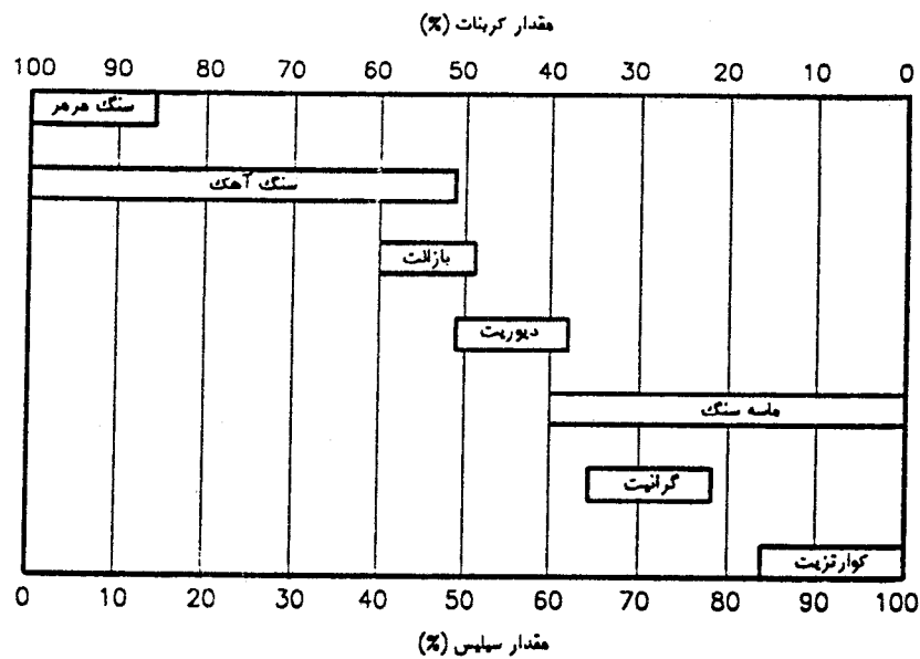
شکل ۲-۱۲: طبقه‌بندی مصالح سنگی [۴]
